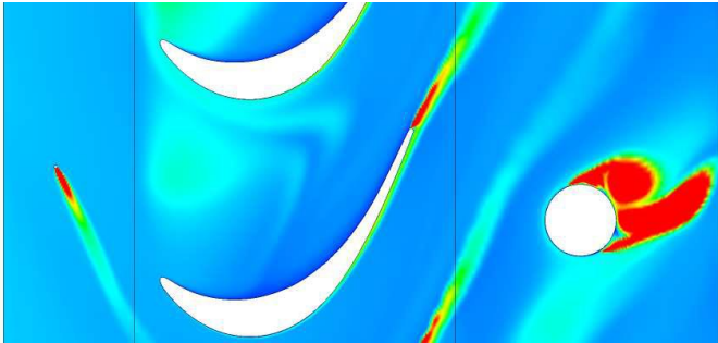
Abbildung 1: TKE innerhalb einer Schaufelpassage
