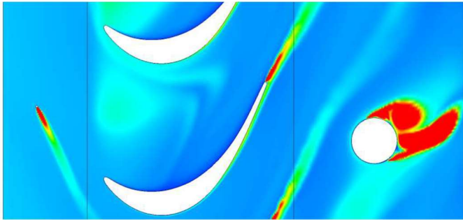
Abbildung 1: TKE innerhalb einer Schaufelpassage
